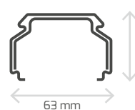
41 mm TRILUX E-LINE
