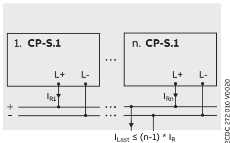
Parallelbetrieb, Redundanz (n ≤ 3)
