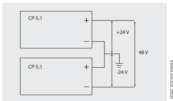
Anschlussplan für +/- 24- oder 48 V-DC-Ausgangsspannung
