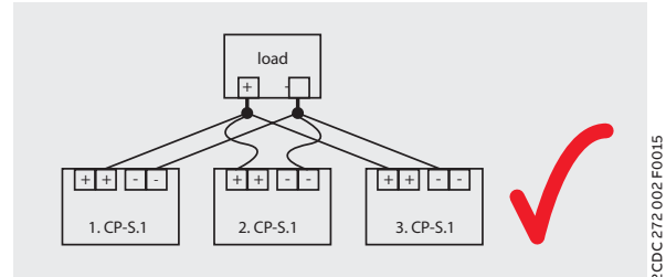
Ordnungsgemäße Verdrahtung zur Leistungserhöhung
