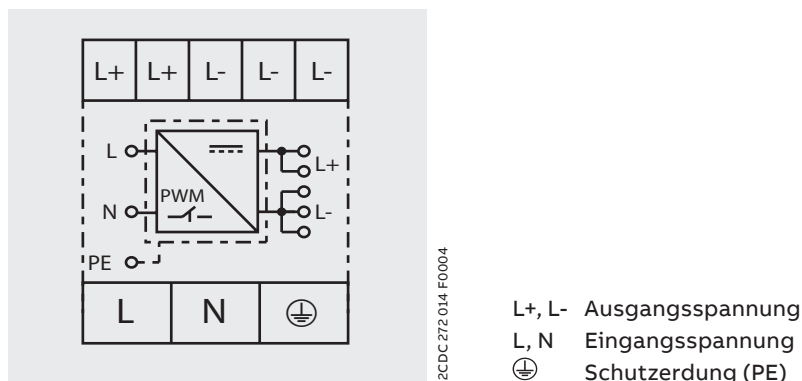
Schaltbild
