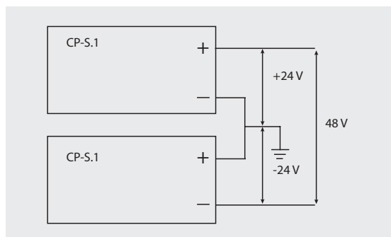
Anschlussplan für +/- 24- oder 48 V-DC-Ausgangsspannung
