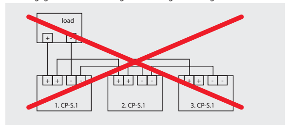
Falsche Verdrahtung zur Leistungserhöhung
