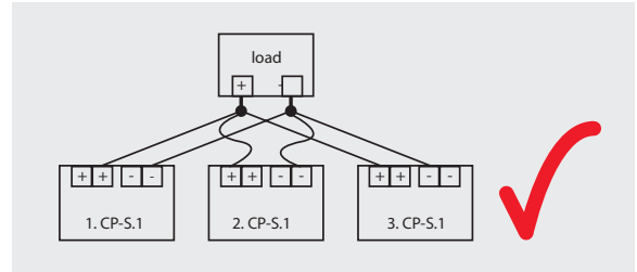
Ordnungsgemäße Verdrahtung zur Leistungserhöhung
