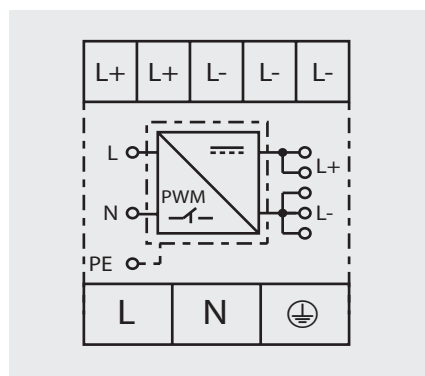
Schaltbild
