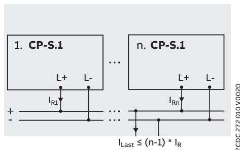
Parallelbetrieb, Redundanz ( n \leq 3 )
