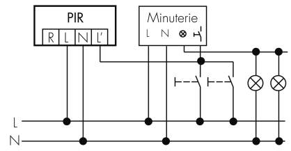
Impulsbetrieb an Treppenhausautomat
