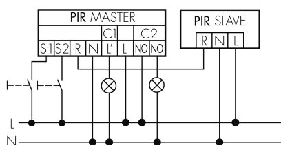
Master-Slave-Betrieb
