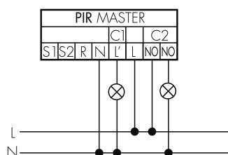
Normalbetrieb
