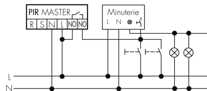
Impulsbetrieb an Treppenhausautomat
