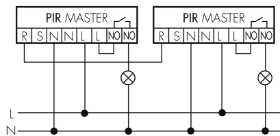
Master-Master-Betrieb
