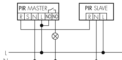
Master-Slave-Betrieb
