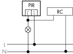
Normalbetrieb mit RC-Glied
