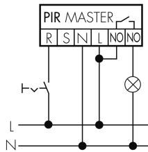
Master-Slave-Betrieb
