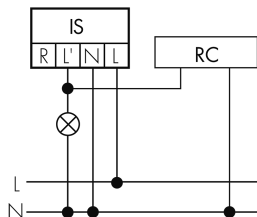
Normalbetrieb mit RC-Glied
