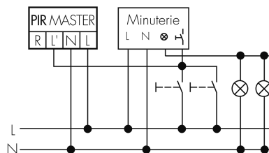
Impulsbetrieb an Treppenhausautomat
