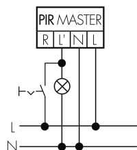
Betrieb mit Drehschalter «Hand - 0 - Automat»
