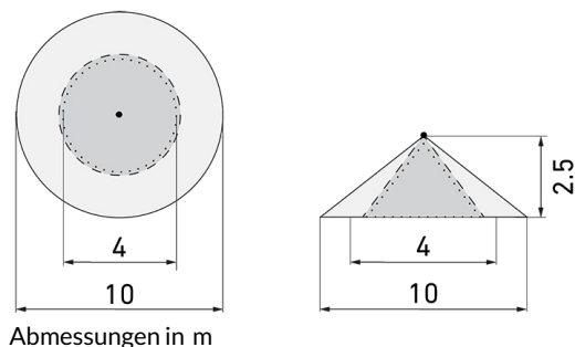
links: Aufsicht, rechts: Seitenansicht
