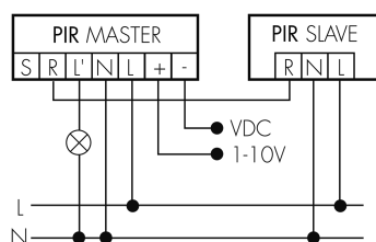
Master-Slave-Betrieb
