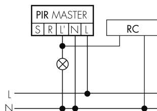
Normalbetrieb mit RC-Glied
