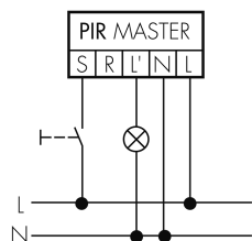
Betrieb mit Drehschalter «Hand - 0 - Automat»
