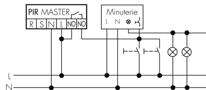
Impulsbetrieb an Treppenhautautomat
