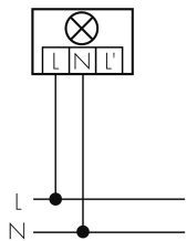
Parallelbetrieb
