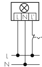
Dauerlichtbetrieb mit externem Schalter
