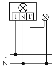
Normalbetrieb mit externer Leuchte
