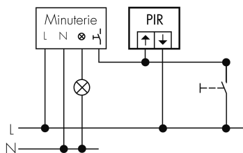
4-Leiter-Schaltung
