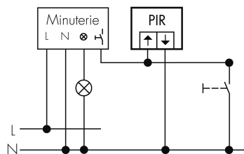
3-Leiter-Schaltung
