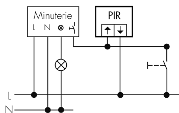
4-Leiter-Schaltung
