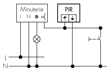
3-Leiter-Schaltung
