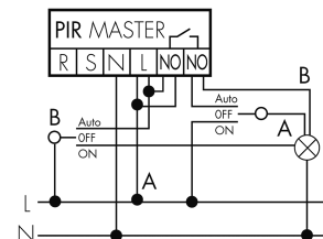
Betrieb mit Drehschalter «Hand - 0 - Automat»
