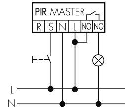
Impulsbetrieb an Treppenhautautomat
