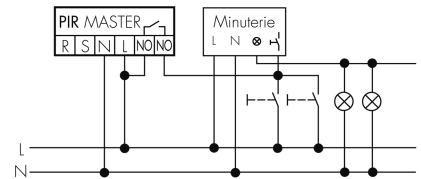
Impulsbetrieb an Treppenhautautomat
