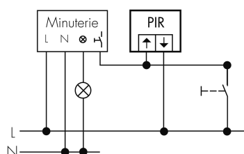
4-Leiter-Schaltung
