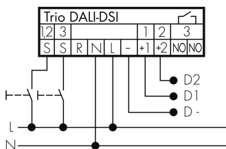
Normalbetrieb mit externem Taster, 2 Taster Modus
