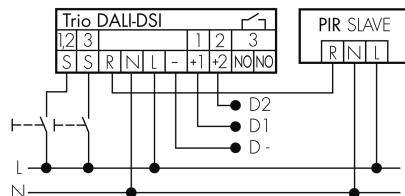
Master-Slave-Betrieb mit externem Taster, 2 Taster Modus
