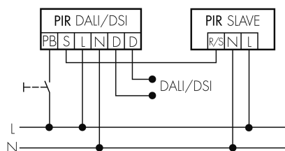
Master-Slave-Betrieb mit externem Taster
