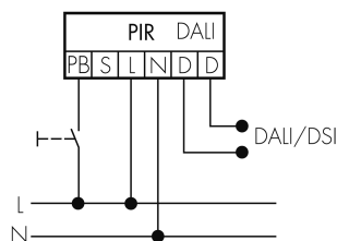
Normalbetrieb mit externem Taster
