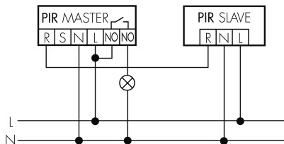
Fonctionnement Master-Slave
