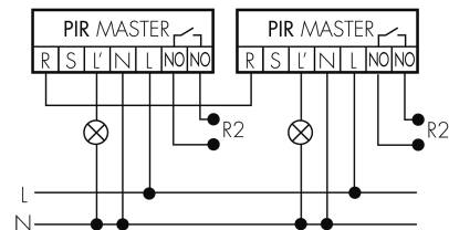
Fonctionnement normal avec circuit RC
