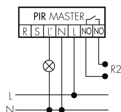
Fonctionnement avec interrupteur rotatif «Manuel - 0 - Automatique»
