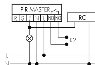
Fonctionnement normal avec circuit RC
