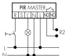
Fonctionnement Master-Slave
