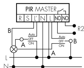
Fonctionnement avec interrupteur rotatif «Manuel - 0 - Automatique»
