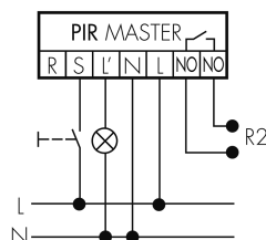
Fonctionnement normal avec bouton externe
