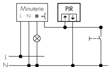
Raccordement 3 fils
