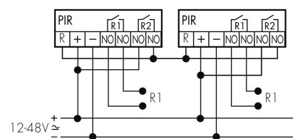
Fonctionnement Master-Master
