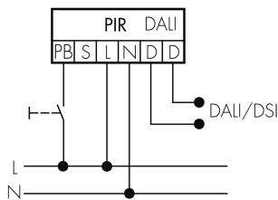
Fonctionnement normal avec bouton externe
