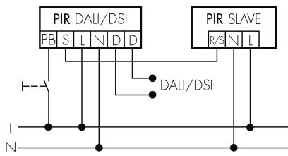
Fonctionnement Master-Slave avec bouton externe
