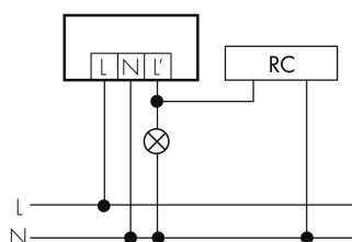
Funzionamento normale con filtro RC
