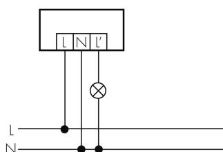
Funzionamento normale
