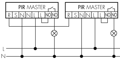
Funzionamento Master-Master
