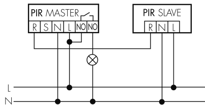
Funzionamento Master-Slave
