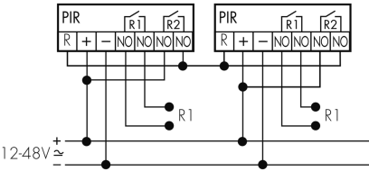
Funzionamento Master-Master
