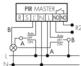
Funzione con commutatore rotativo «Manuale - 0 - Automatico»
