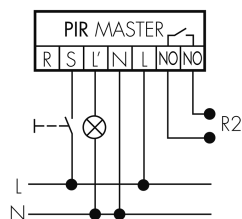
Funzionamento normale con tasto esterno
