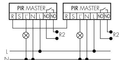
Funzionamento normale con filtro RC
