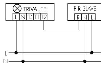
Funzionamento Master-Slave
