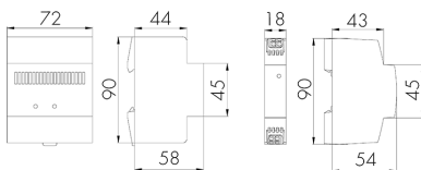
Dimensioni in mm
