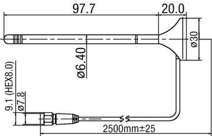
fig. 1. Abmessungen (mm)
