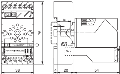
fig. 2. Abmessungen (mm)
