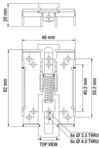
fig. 1. Abmessungen (mm)
