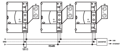
Anschlusschema
