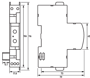
Maßzeichnung Gruppenansicht
