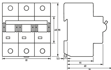
Maßzeichnung Gruppenansicht
