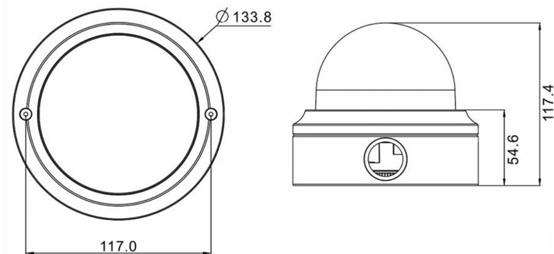
Fig. 1: 4K (8MP) Vandal Fixed Dome Analytics Camera: Tutte le misurazioni in mm
