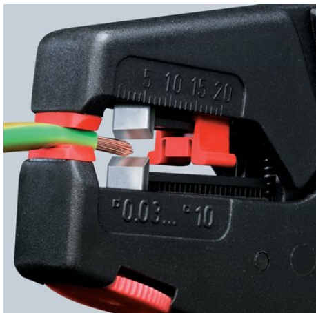
12 40 200: Spelatura precisa senza danneggiamento del conduttore
