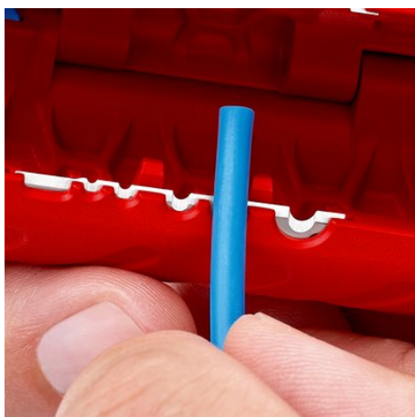
90 22 02 SB: l'aide au positionnement pratique simplifie l'insertion de câbles simples à dénuder
