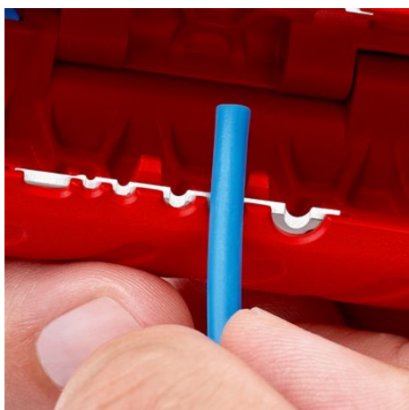
90 22 02 SB: Pratico posizionatore per facilitare l'inserimento di conduttori singoli da spelare
