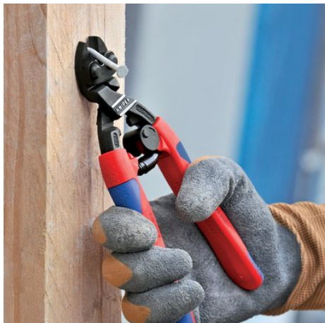
20° gewinkelter Kopf mit einseitiger Lasche und Seitenschnitt zum bündigen Schneiden, mit Freiraum zum Greifen
