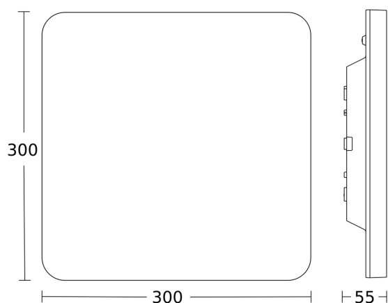
Disegno tecnico
