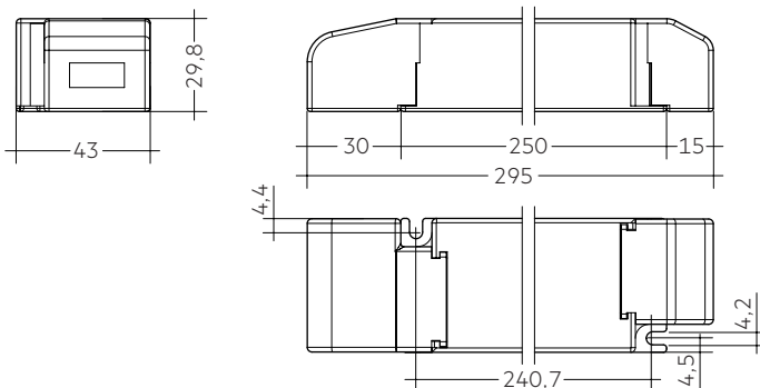
Mit Zugentlastung
