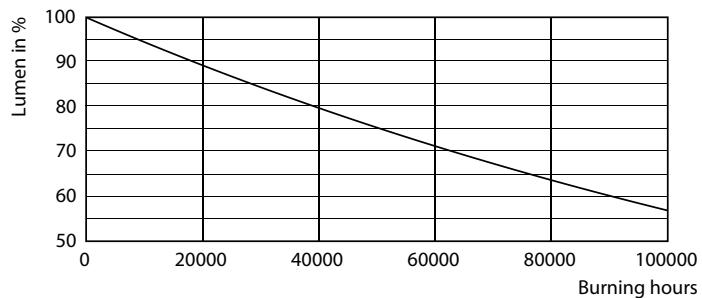
Lumen Maintenance Diagram - MAS LEDtube VLE UN 1500mm UO 23W865
