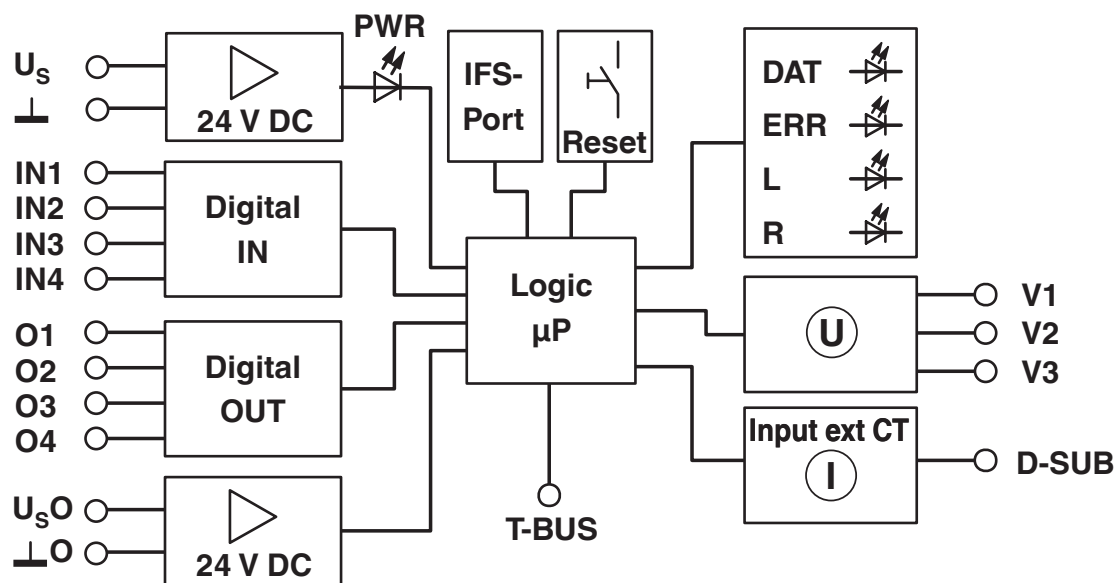
Schéma fonctionnel
